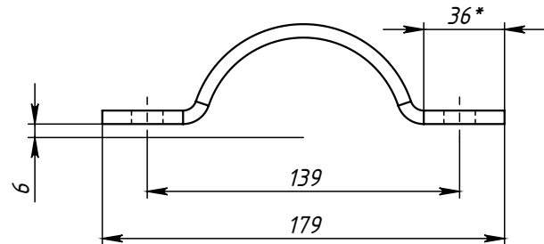
Поз.4 (Полухомут)
