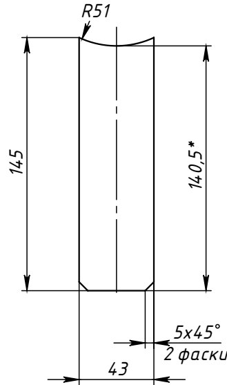
Поз.3 (Ребро)
